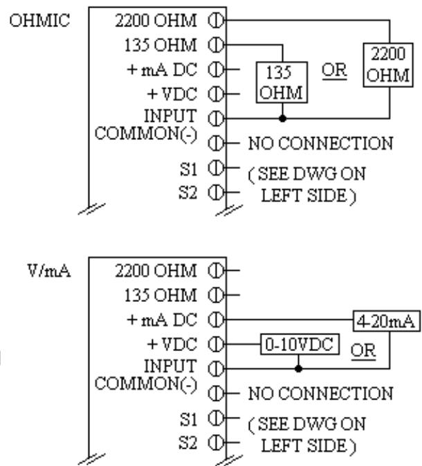
Wiring Diagrams: Inputs
